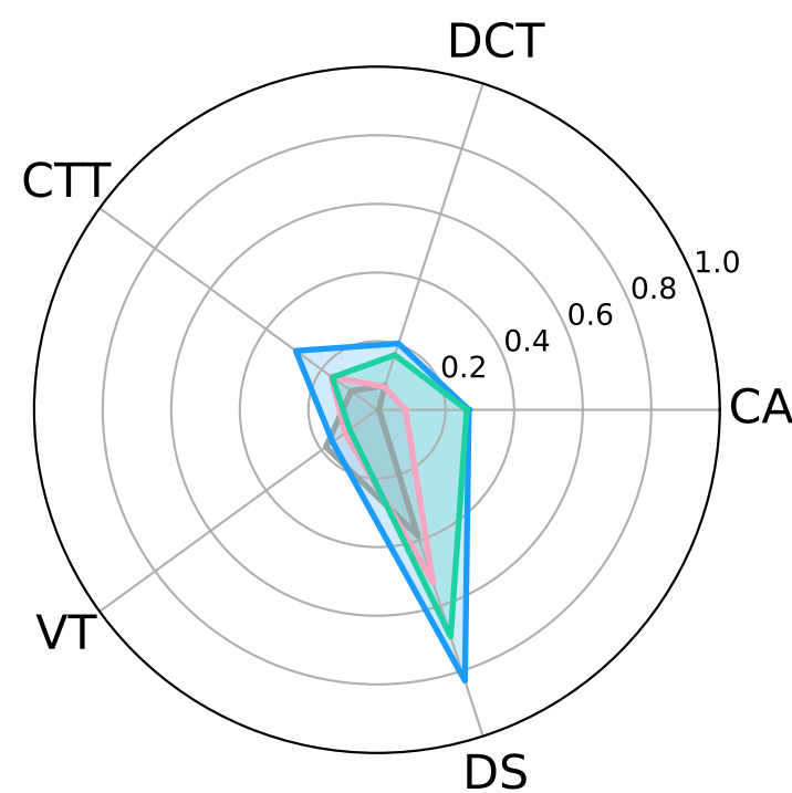
(a) LLaMA-2/3
